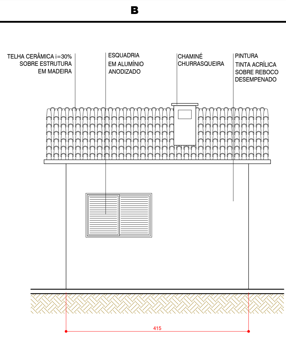
O7 ELEVACÃO 1:50
