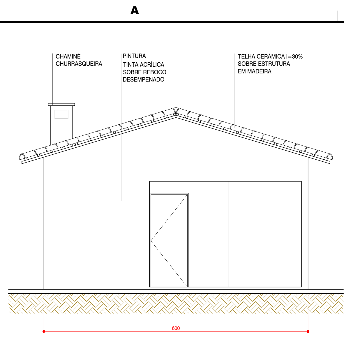
O6 ELEVACÃO 1:50
