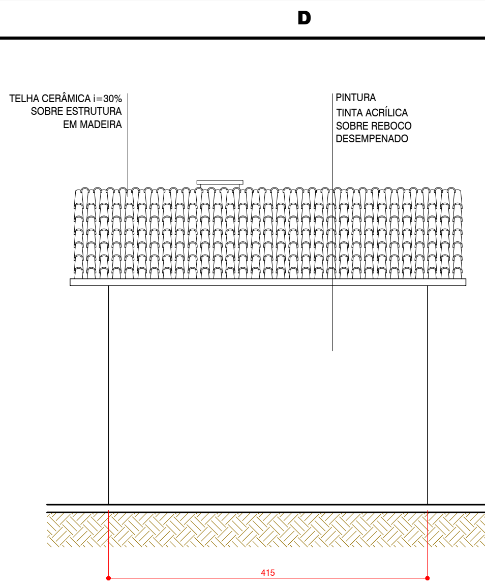
O9 ELEVACÃO 1:50
