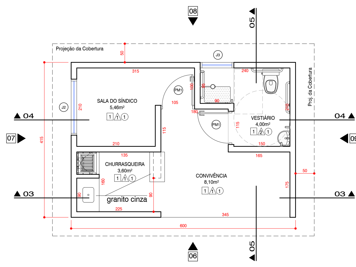
O1 PLANTA PAV. TÉRREO 1:50
