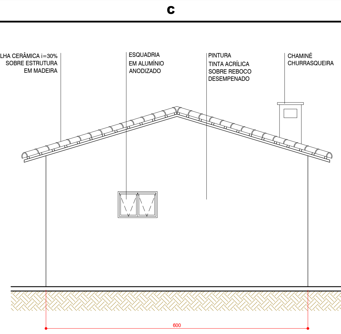
O8 ELEVACÃO 1:50
