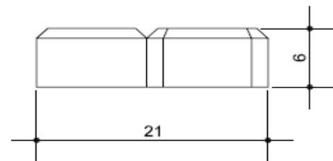
ELEVAÇÃO
