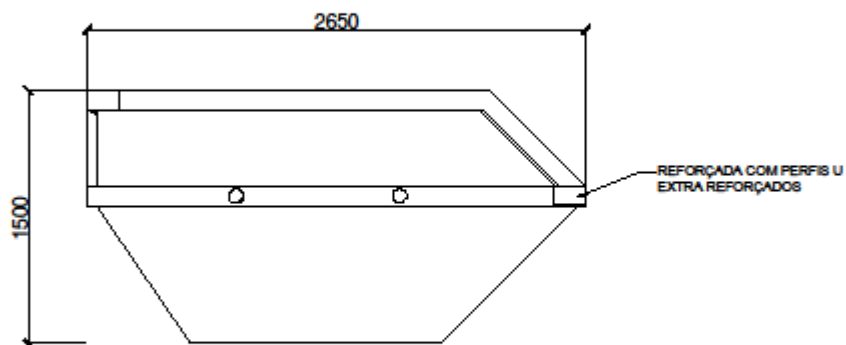
VISTA LATERAL
