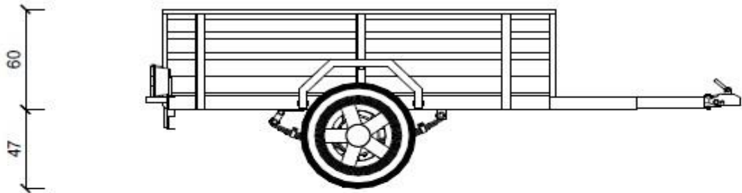
VISTA LATERAL
