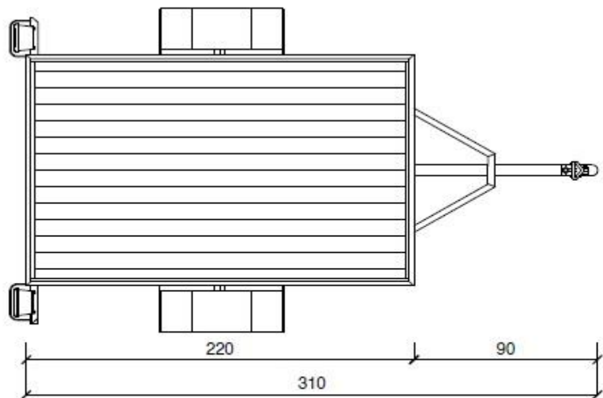
VISTA SUPERIOR
