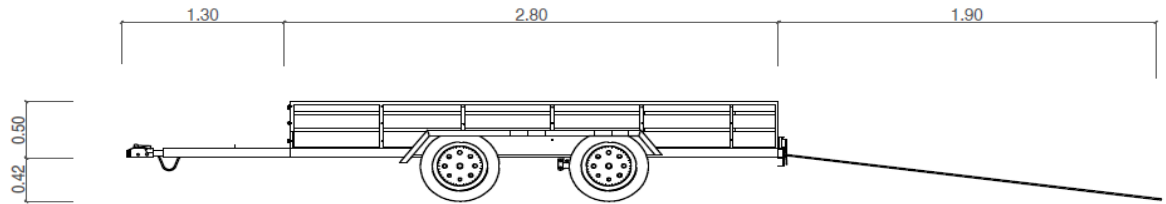
VISTA LATERAL
