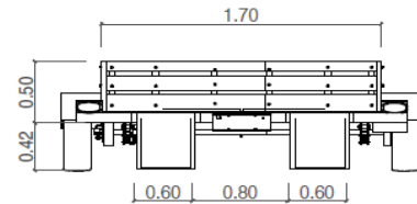
VISTA TRASEIRA
