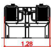
02 1:50 ELEVÇÃO
