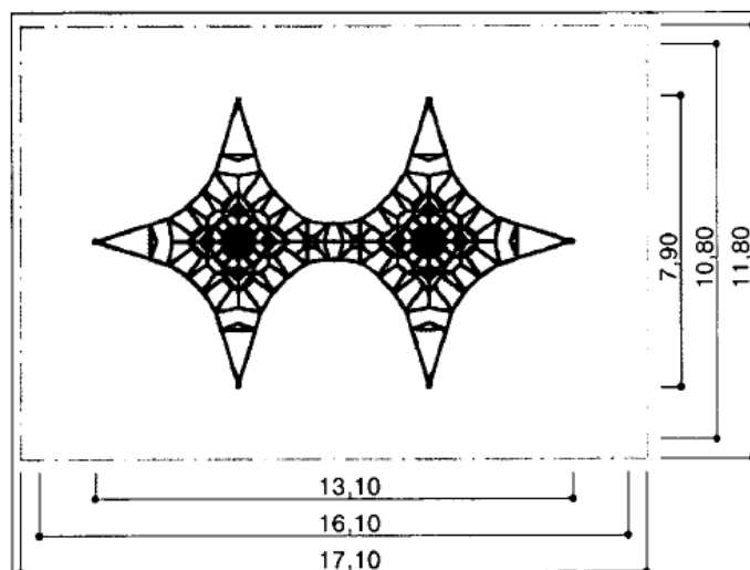
03 _____ S/ESCALA PLANTA
