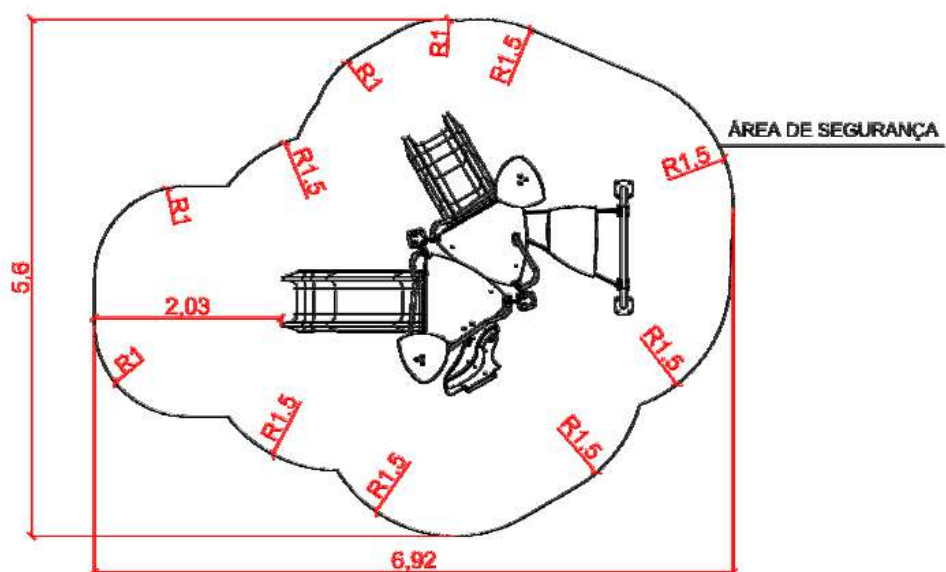
01 _____ 1:75 PLANTA
