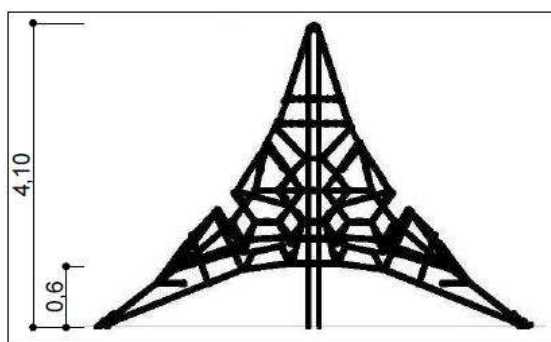
02 _____ S/ESCALA ELEVAÇÃO
