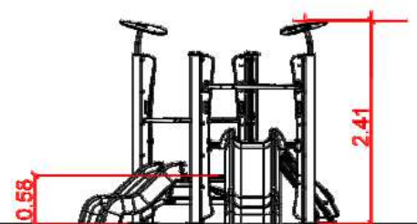
04 _____ 1:75 ELEVÇÃO
