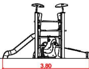
03 _____ 1:75 ELEVÇÃO
