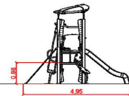
04 ELEVAÇÃO
