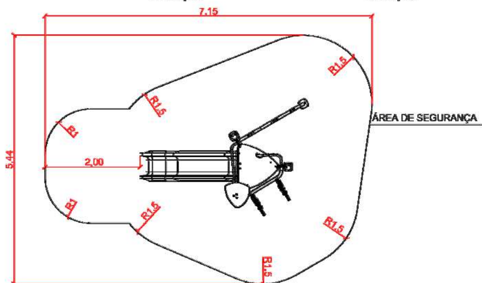
01 PLANTA 1:75
