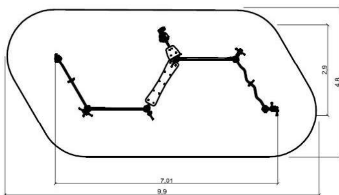
01 1:100 PLANTA
