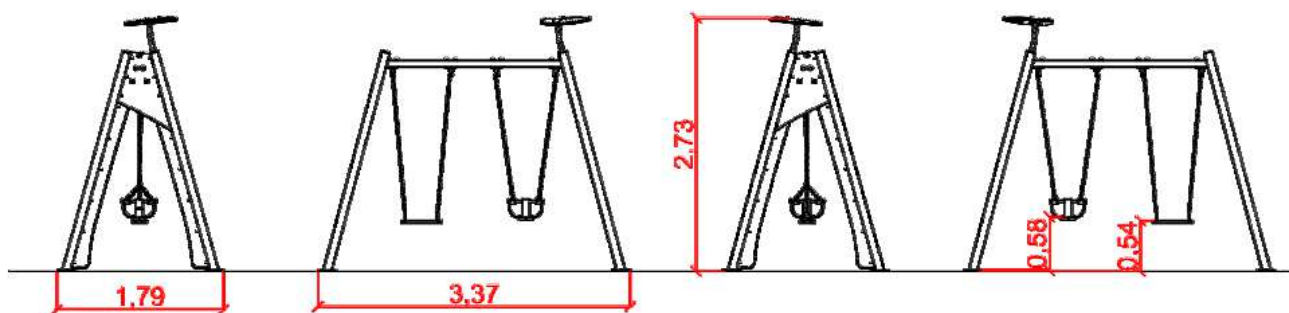
02 1:75 ELEVAÇÃO
