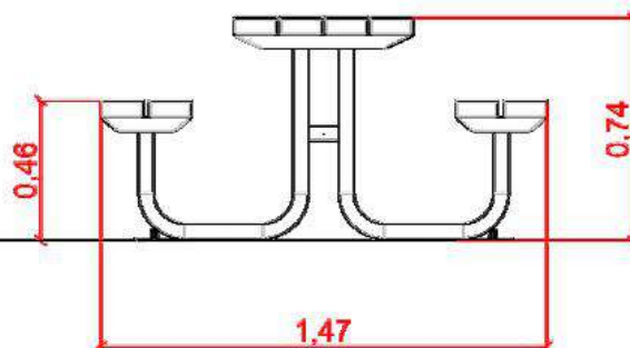
03 _____ 1:25 ELEVAÇÃO
