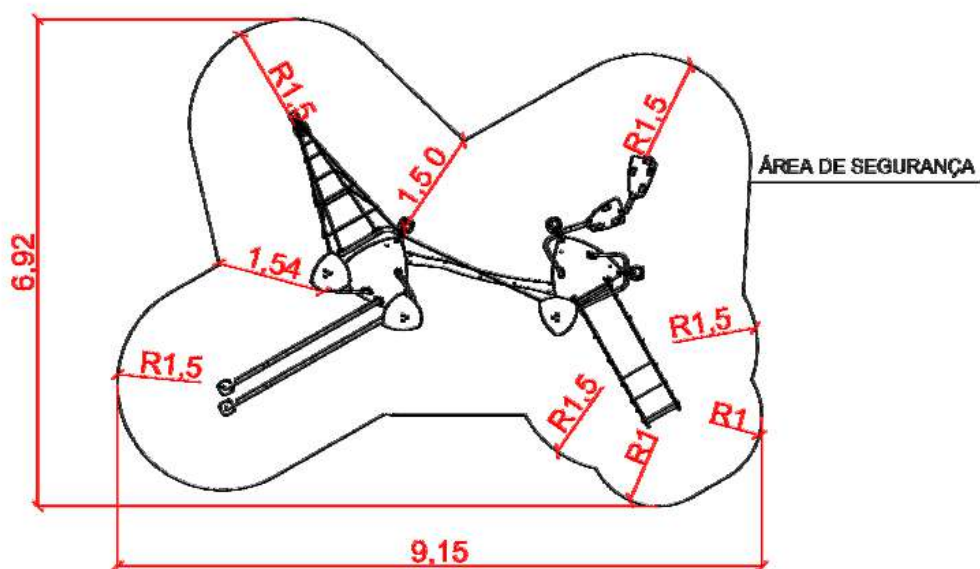
01 _____ 1:100 PLANTA
