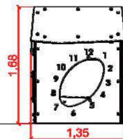
05 1:50 ELEVAÇÃO
