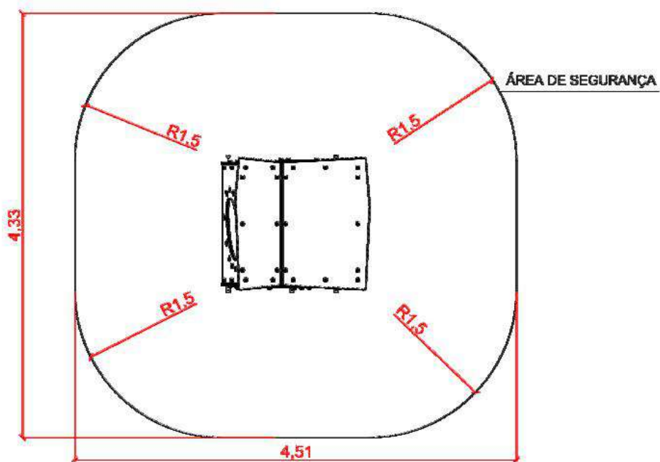
01 1:50 PLANTA
