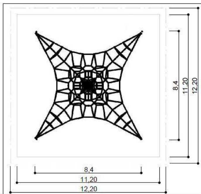
03 _____ S/ESCALA PLANTA
