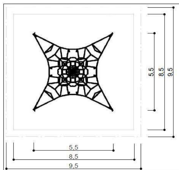
03 _____ S/ESCALA PLANTA
