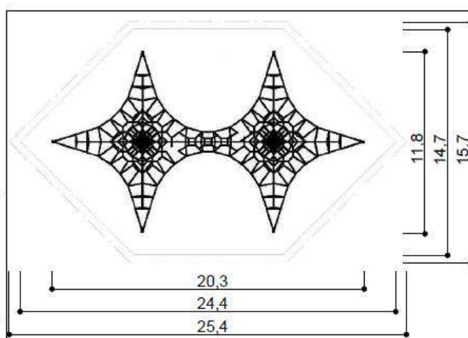
03 _____ S/ESCALA PLANTA
