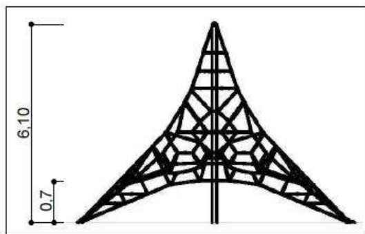
02 _____ S/ESCALA ELEVAÇÃO
