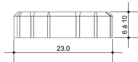
ELEVAÇÃO 1
