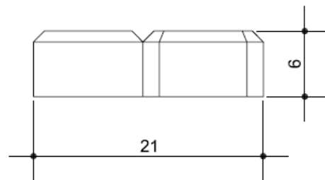
ELEVAÇÃO
